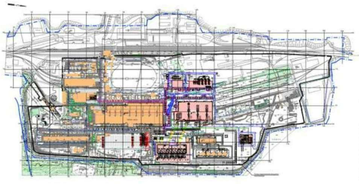
Рисунок 1.10. В.4.2. Генеральный план
