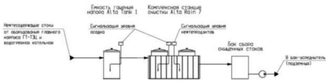
Принципиальная схема установки очистки нефтесодержащих стоков главного корпуса ГТ-ТЭЦ и водогрейной котельной
