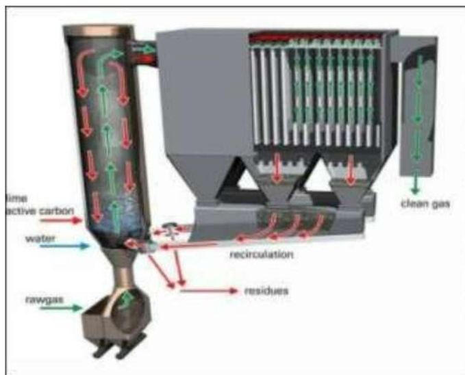
Рисунок 2.7. Система сухой очистки дымовых газов Turbo-CDS
