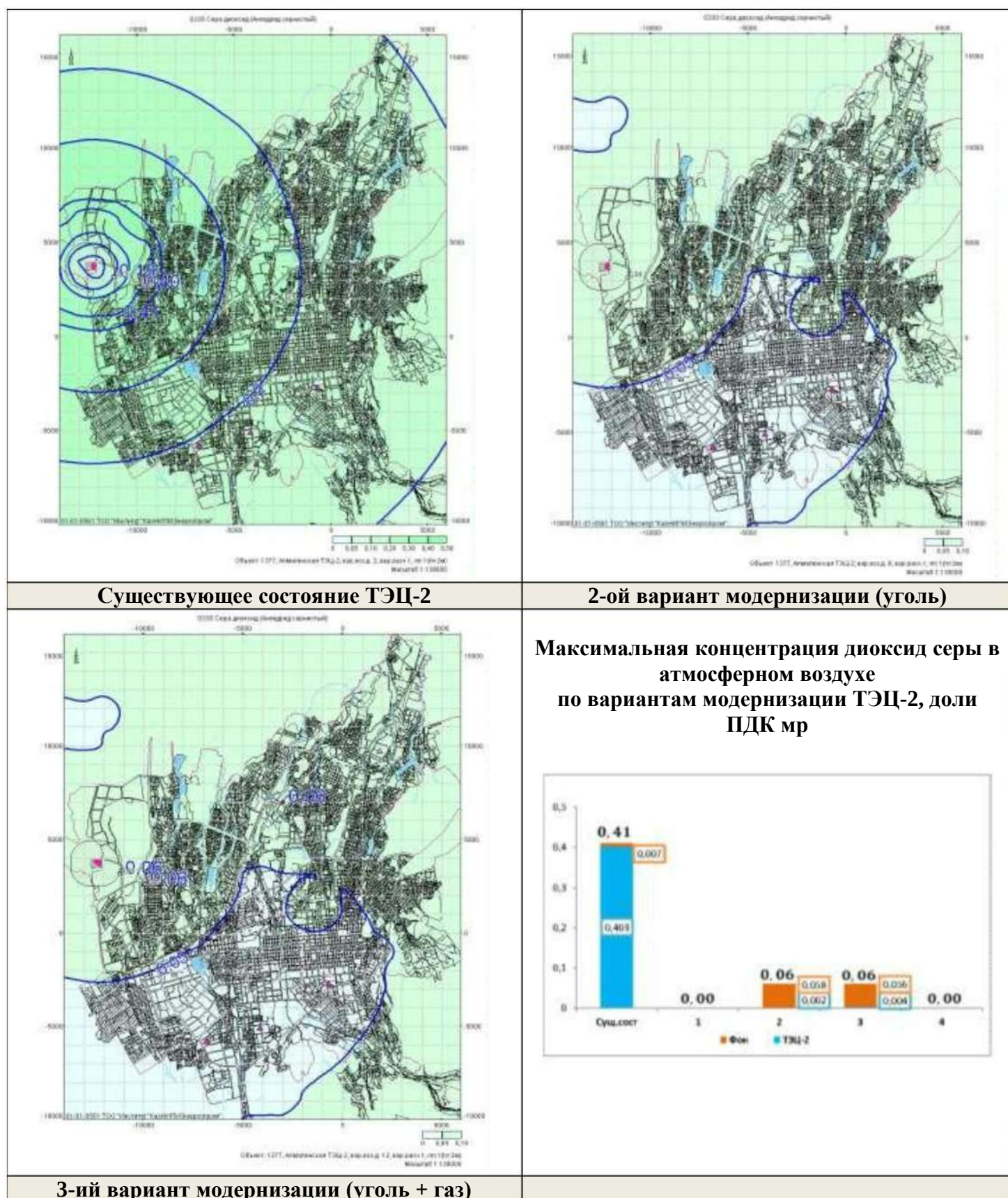
Рисунок 2.18. Расчетное загрязнение выбросами \text{SO}_2
