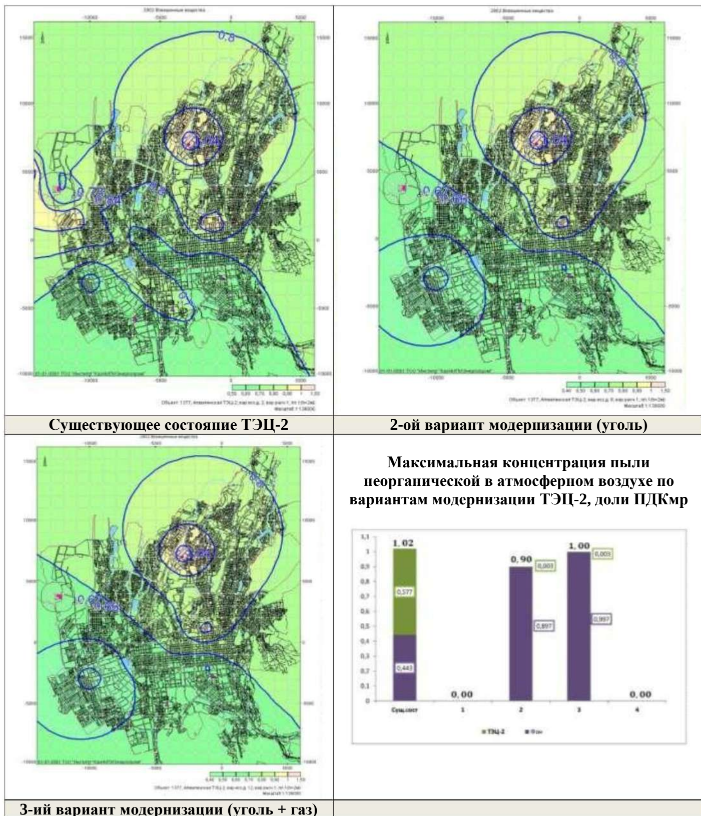
Рисунок 2.19. Расчетное загрязнение атмосферы выбросами пыли неорганической (с учетом фона ПДК= 0,5 мг/м 3 )
