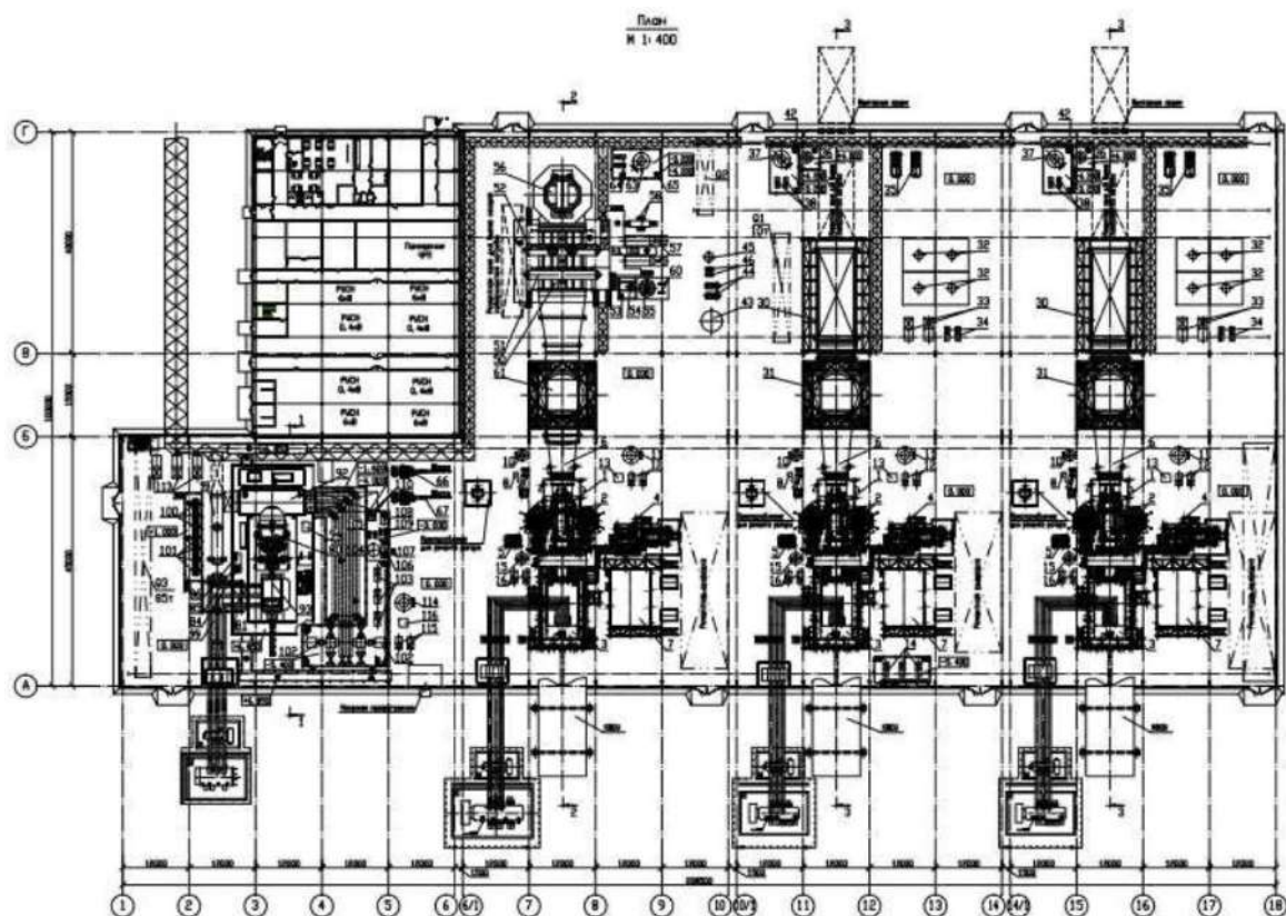
Рисунок 1.8. В.4.2. Компоновка главного корпуса ГТ-ТЭЦ
